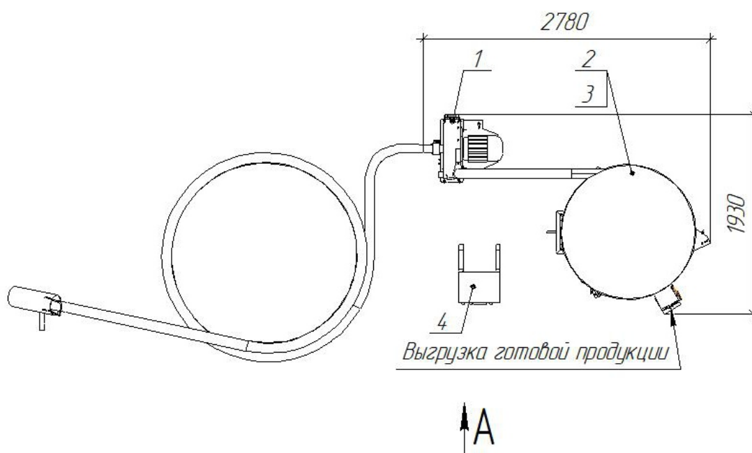
Экспликация оборудования
